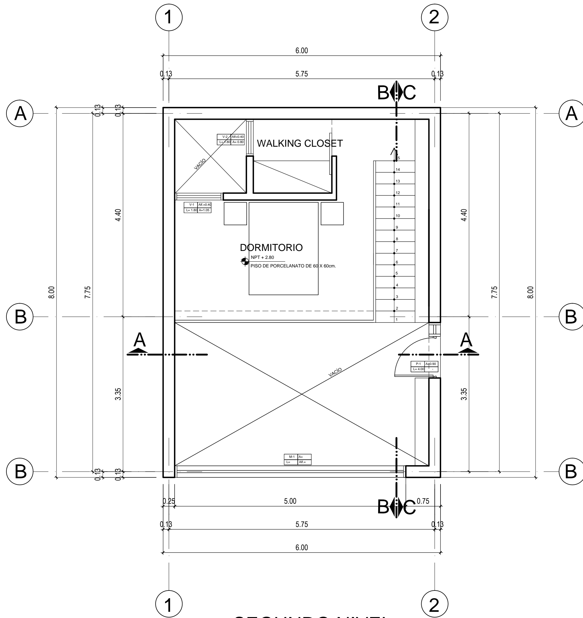
SEGUNDO NIVEL ESCALA 1:50
