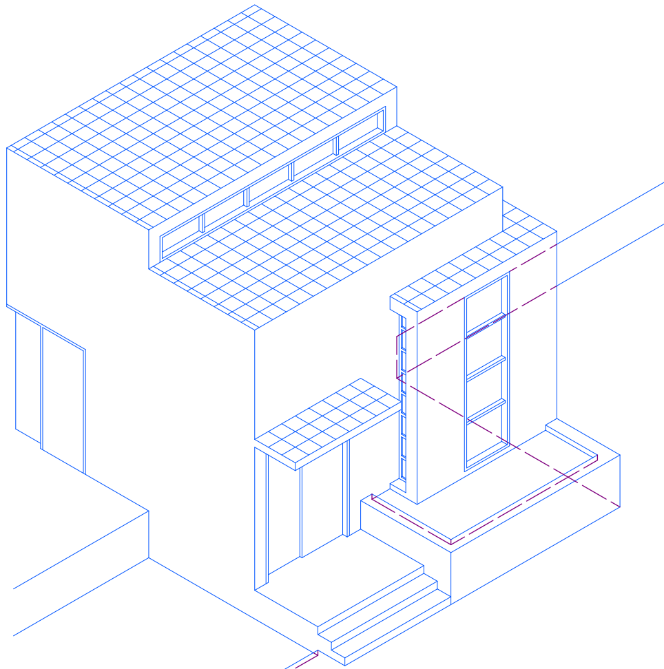
ISOMETRÍA 01, ESCALA 1/100
